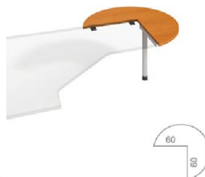
GP 21 P \varnothing 100 \times 75,5 \times (60 \times 60)
